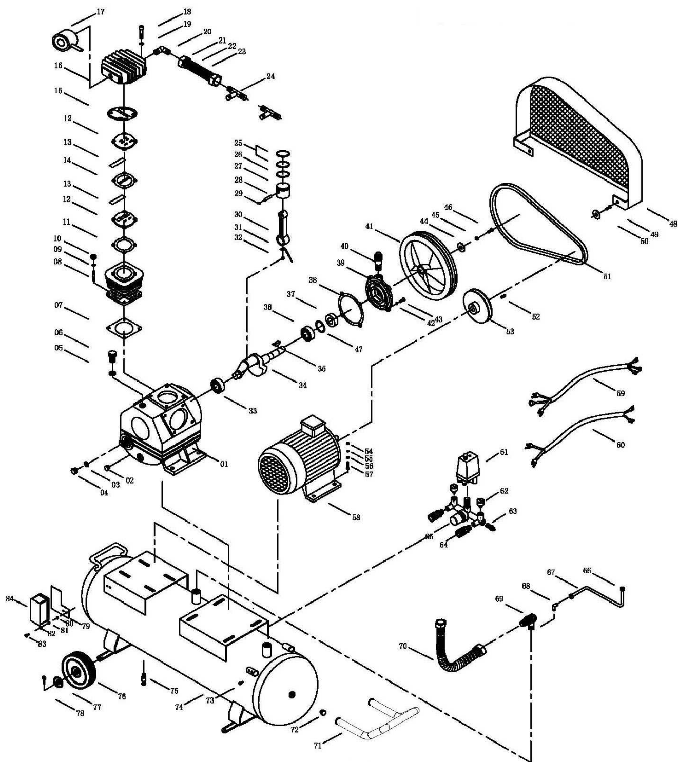
Рисунок 2. TORNADO 140
